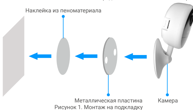
Рисунок 1. Монтаж на подкладку
